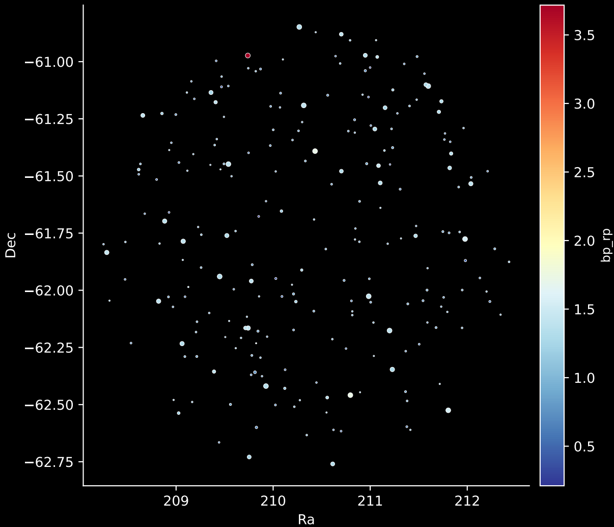
GALAH DR4 Field: [7193] Stars: 234
