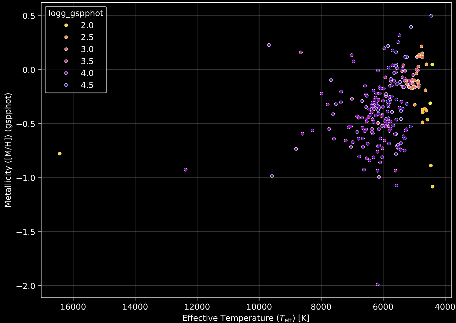
GALAH DR4 Field: [7193] Stellar Population Parameters (n= 234)
